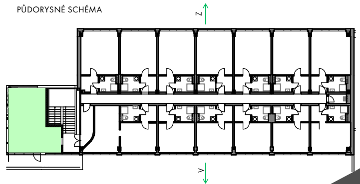
PŮDORYSNÉ SCHÉMA
